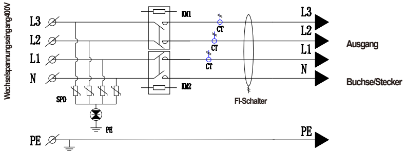
Abb. 14-1. Hauptstromkreis
