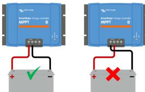
Beispiele für richtige und falsche (vertauschte) Batteriepolartität.
