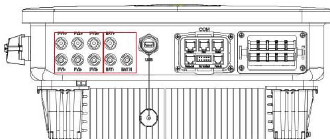
Abbildung 5-6: PV-Eingänge
