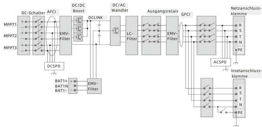
Abbildung 2-1: Schematische Darstellung
