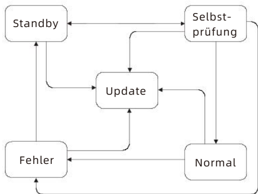
Abbildung 2 - 2 : Betriebsmodi
