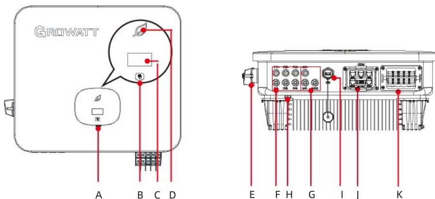
Abbildung 3- 3: Geräteansicht
