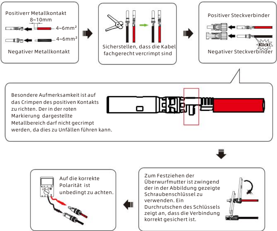
Abbildung 5-7: Vorbereitung der PV-Eingangskabel
