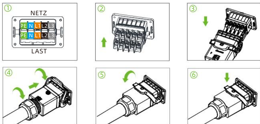
Abbildung 5-5: Endgültige Fertigstellung
